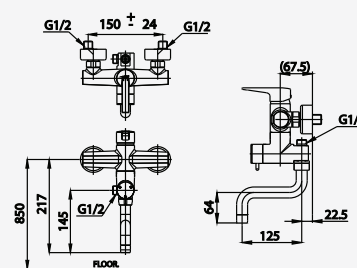
■ CT5102A Lever Handle Concealed Mixer Stop Valve with Diverter (3 Ways) ก๊อกผสมยื่นอาบน้ำพร้อมตัวก๊อกลงพื้น (เกลี่ยวนบน)
