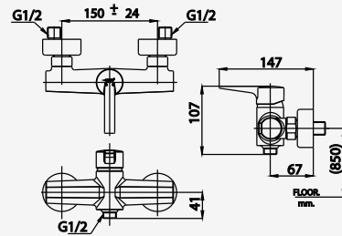
■ CT2264A Lever Handle Exposed Shower Mixer ก๊อกผสมยื่นอาบน้ำแบบก้านโยก
