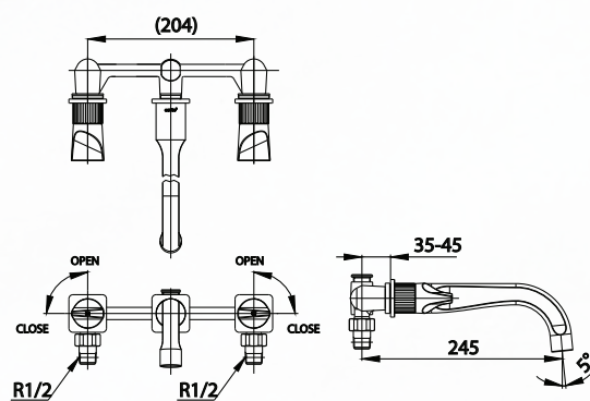
■ CT2283C44 3 Hole 8" Basin Mixer Faucet wall-mounted ก๊อกผสมอ่างล้างหน้า เซ็นเตอร์ 8 ชนิดติดผนัง
