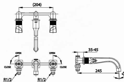
■ CT2283C45 3 Hole 8" Basin Mixer Faucet wall-mounted ก๊อกผสมอ่างล้างหน้า เซ็นเตอร์ 8 ชนิดติดผนัง
