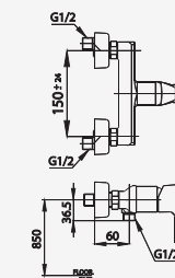
■ CT2205A Lever Handle Exposed Shower Mixer ก๊อกผสมยืนอ่างแบบก้านโยก
