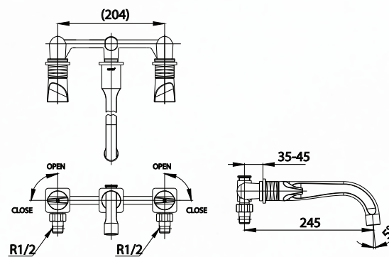
■ CT2283C46 3 Hole 8" Basin Mixer Faucet wall-mounted ก๊อกผสมอ่างล้างหน้า เซ็นเตอร์ 8 ชนิดติดผนัง
